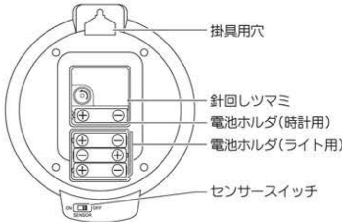
光センサー
